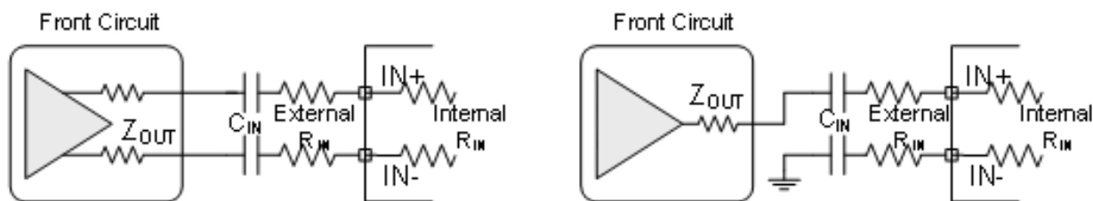
图 1 (1) 差分输入;
