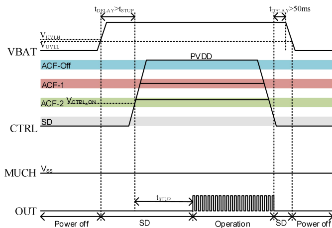
图表 9 利用关断模式减小 Pop 声时序图
