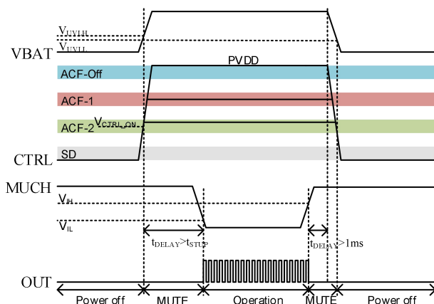
图表 8 利用静音模式减小 Pop 声时序图
